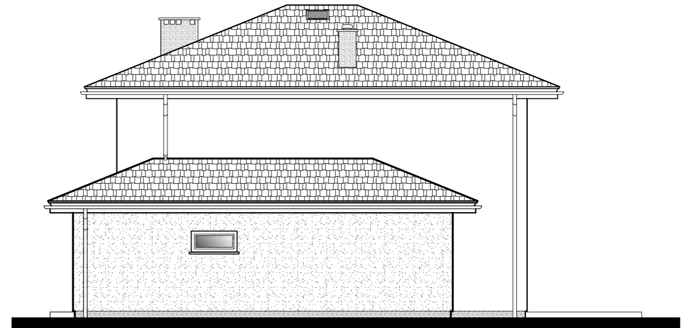
ELEWACJA BOCZNA - PÓŁNOCNA
