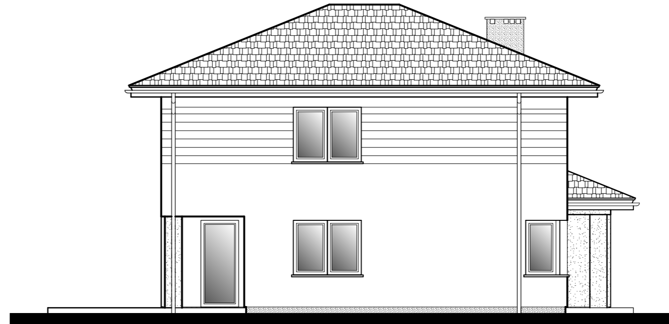
ELEWACJA BOCZNA - POŁUDNIOWA
